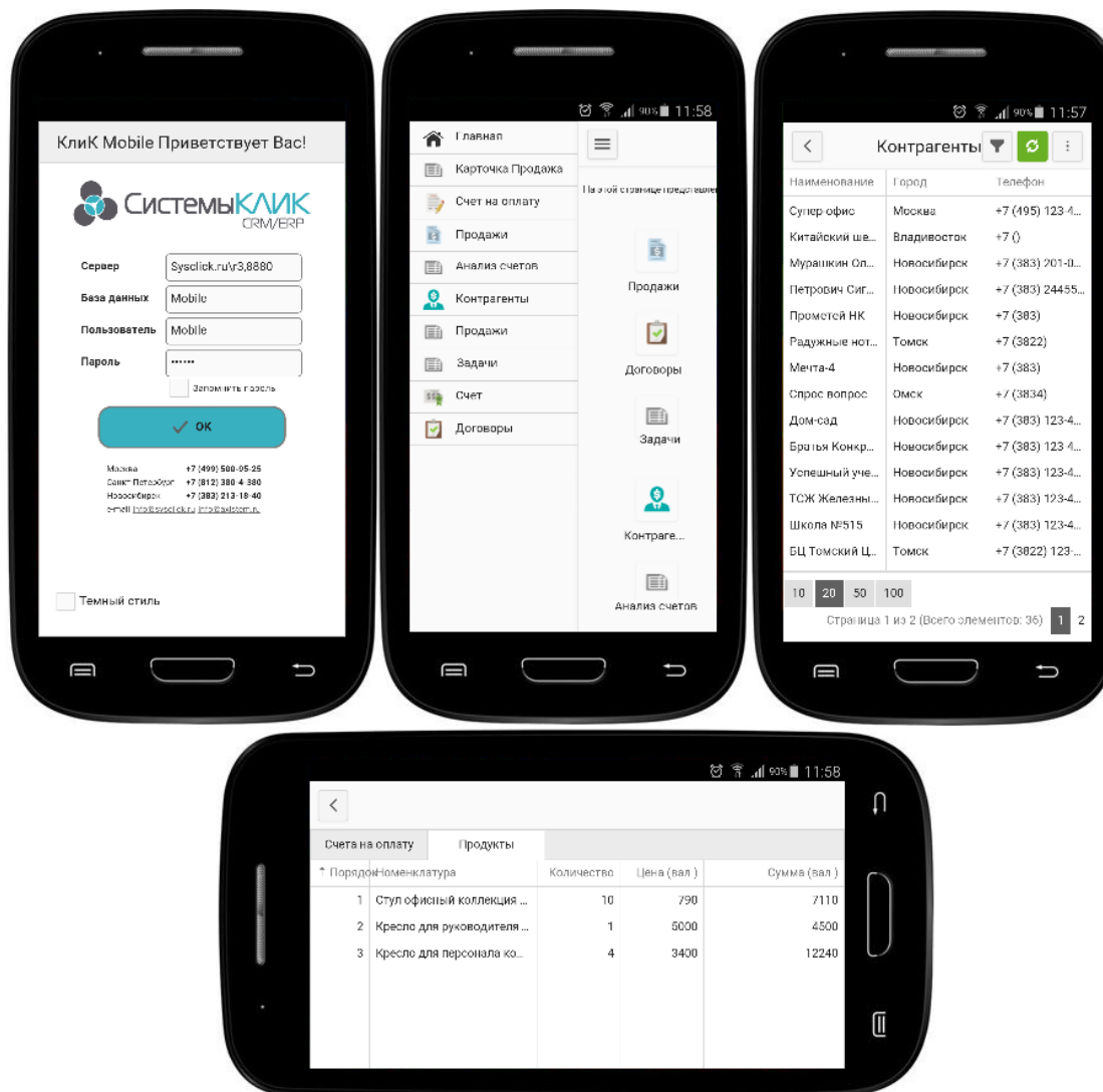
Рисунок 14 Мобильный клиент
