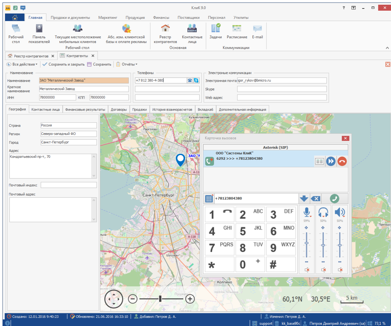
Рисунок 15 Карточка вызова.
