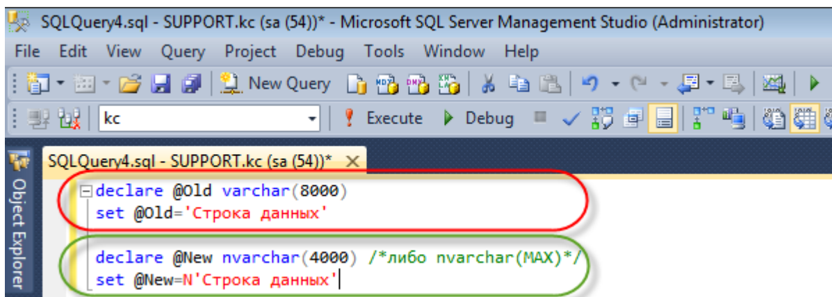
Рисунок 3 Типы данных в Процедурах и Триггерах
