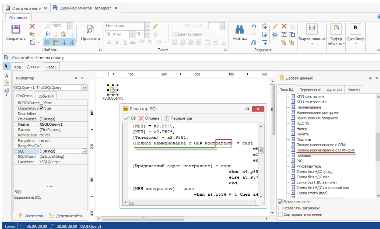
Рисунок 2 Редактор отчета Fast Report, для корректной работы отчета "Счет на оплату" необходимо удалить "рагент" в названии поля (выделен красным).
